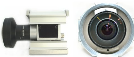
Die Montage garantiert exzellente Wärmeableitung
